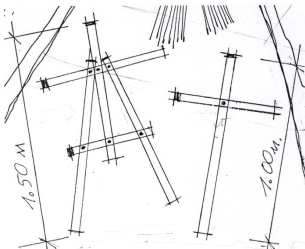
Muoriu karkasu brėžinė
